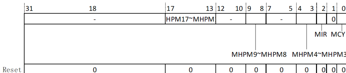
图 12.2: 机器模式计数禁止授权寄存器 (M_COUNTINHIBIT)
