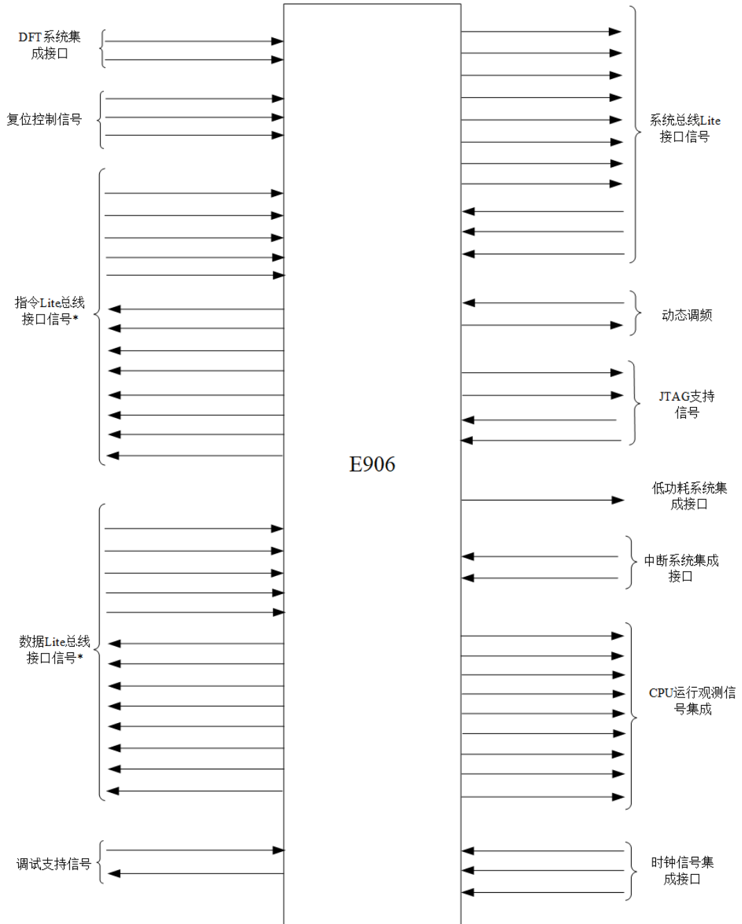
图 2.7: E906 接口总览
