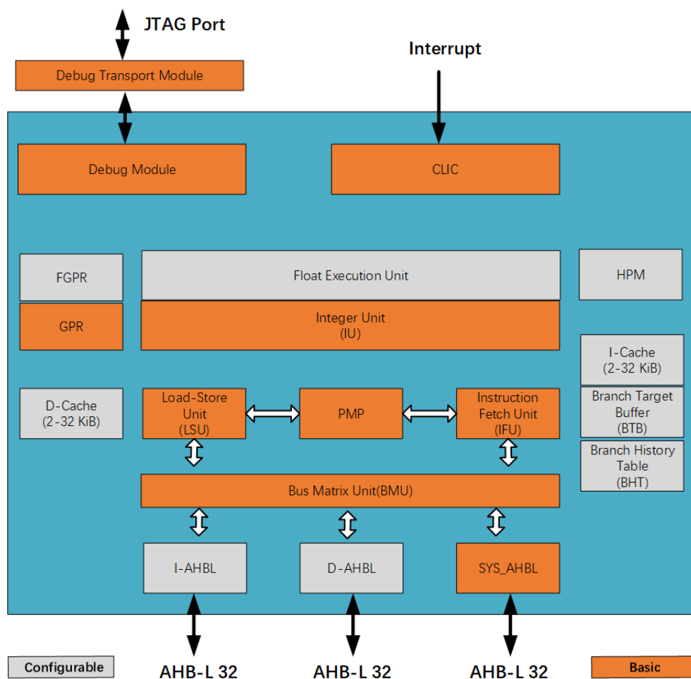
图 2.1: E906 结构图
